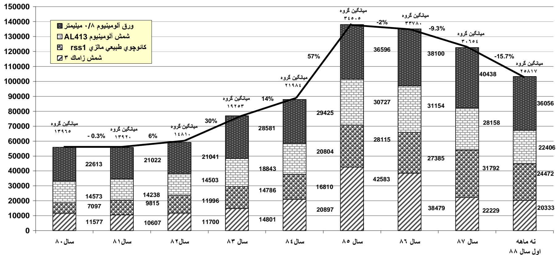
روند تغییرات میانگین قیمت سالیانه گروه سایر مواد پرمصرف درصنعت خودرو به تفکیک طی سالهای ۸۰ تا پایان آذر ۸۸
