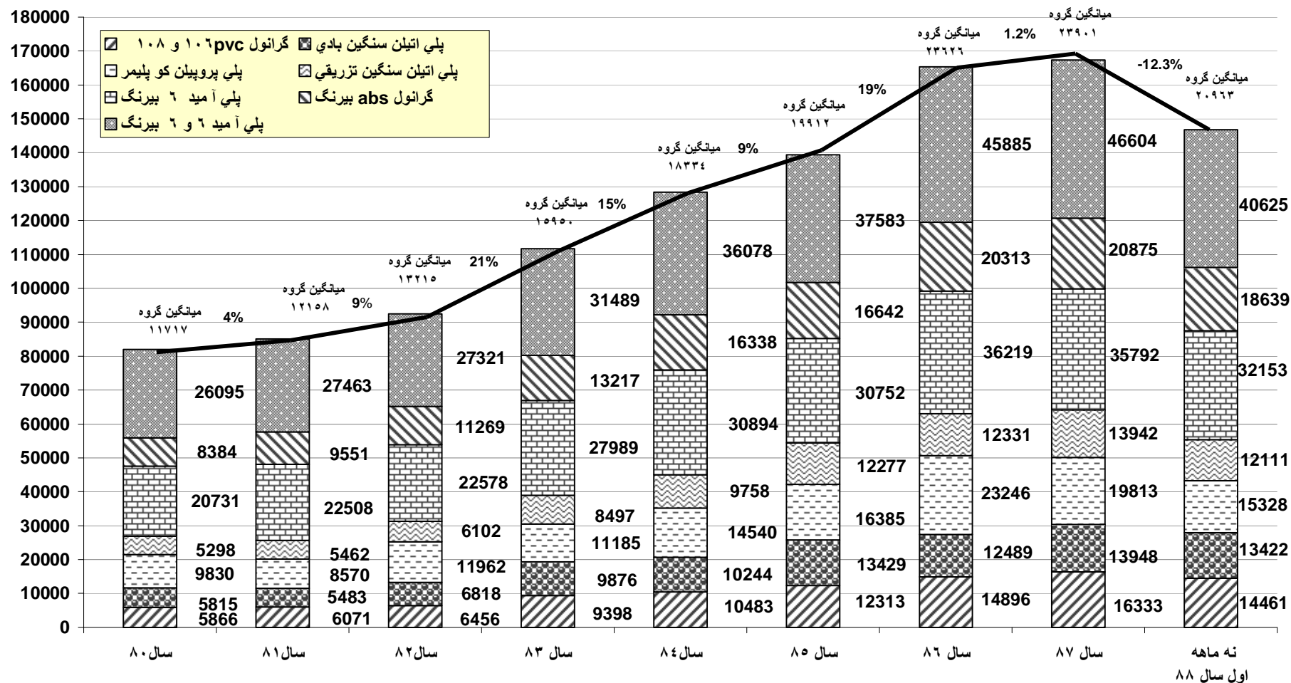
روند تغییرات میانگین قیمت سالیانه عمده ترین مواد پلیمری و پلاستیکی پرمصرف در صنعت خودرو به تفکیک طی سالهای ۸۰ تا پایان آذر ۸۸
